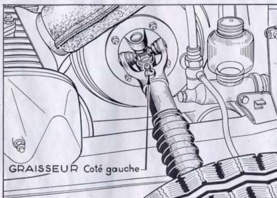
Fig. 14. — (1 graisseur à droite et 1 à gauche)
