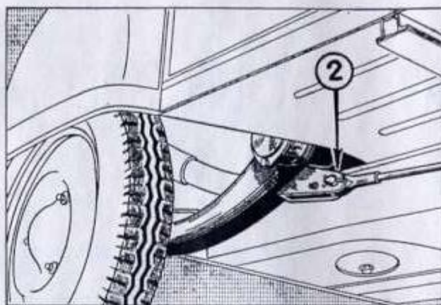
Fig. 18. — Partie arrière (suspension)
