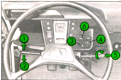
Fig. 22 Commande de signalisation 2 CV6 Spécial 1 - Clignotants droit 2 - Clignotants gauche 3 - Lave-glace 4 - Essuie-glace 5 - Projecteurs et avertisseur sonore 6 - Signal de détresse
