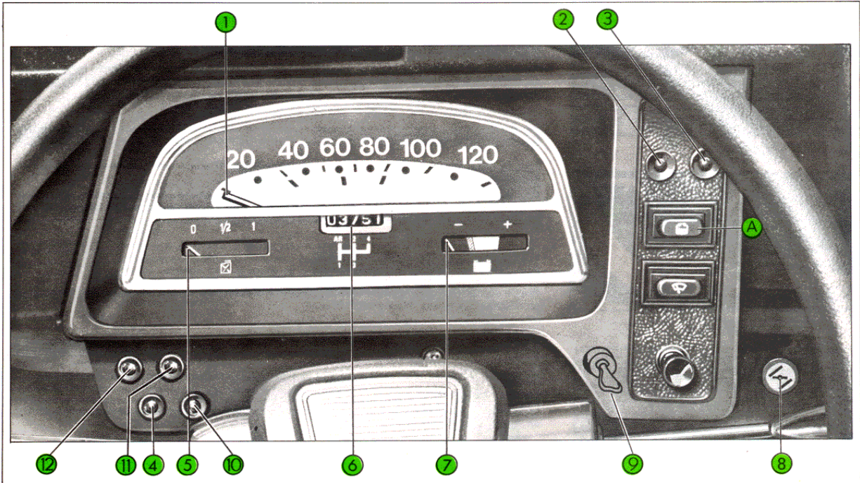
Fig. 10 Poste de conduite; Instruments de bord
