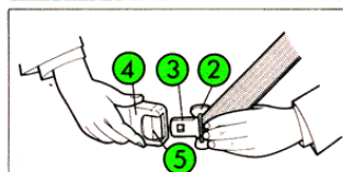
Fig. 14 Ceintures de sécurité avant 1 - Boîtier d'enrouleur 2 - Support pêne de verrouillage 3 - Pêne de verrouillage 4 - Boucle 5 - Poussoir rouge de déverrouillage
