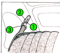
Fig. 15 Ceintures de sécurité arrière 1 - Pêne de verrouillage 2 - Griffe d'accrochage 3 - Support-pêne 4 - Boucle 5 - Boucle de réglage 6 - Poussoir de déverrouillage
