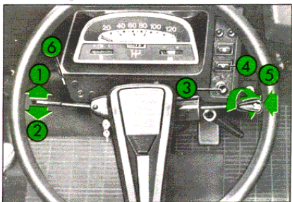
Fig. 23 Commande de signalisation 2 CV6 Charleston 1 - Clignotants droit 2 - Clignotants gauche 3 - Lave-glace 4 - Essuie-glace 5 - Projecteurs et avertisseur sonore 6 - Signal de détresse
