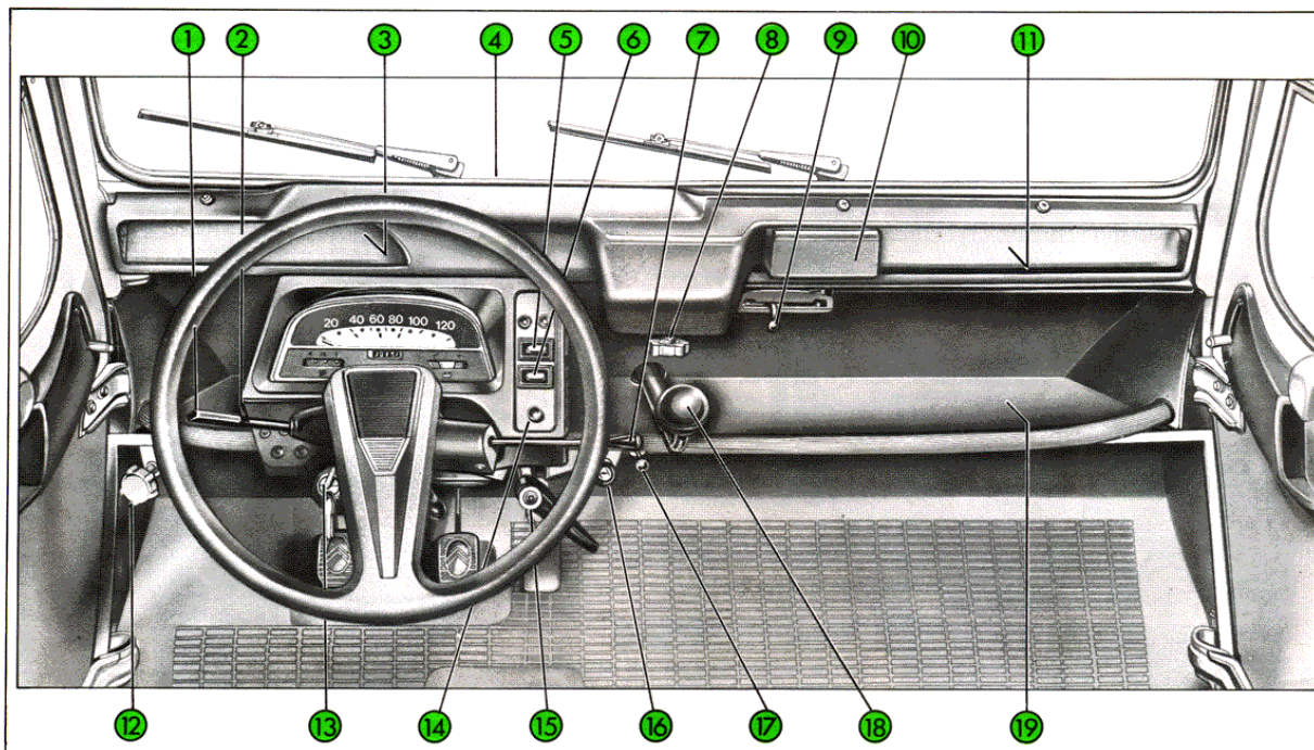
Fig. 8 Poste de conduite : Commandes et accessoires
