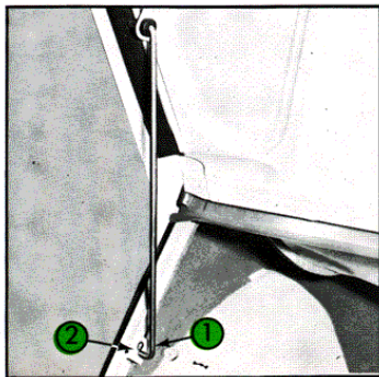
Fig. 4 Porte arrière de coffre 1 - Béquille 2 - Support
