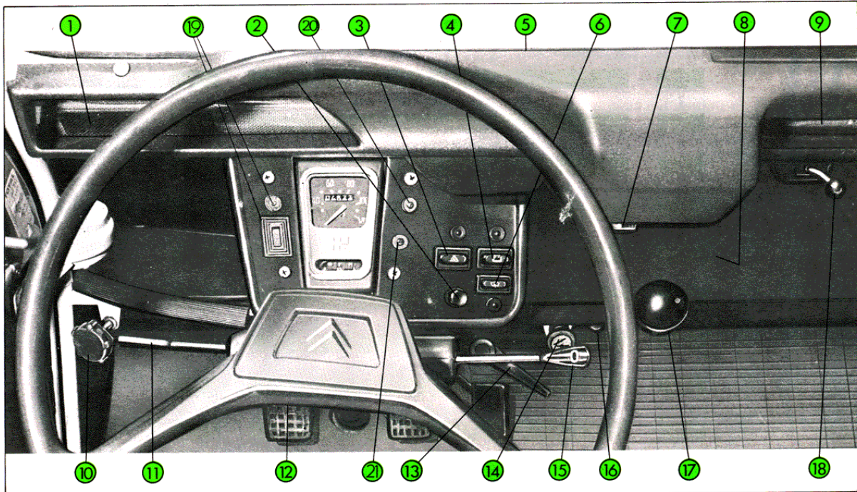
Fig. 7 Poste de conduite: Commandes et accessoires
