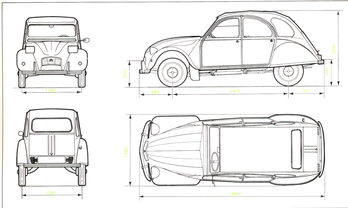
Fig. 3 Cotes d'encombrement
