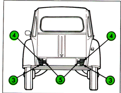
Fig. 5 Eclairage extérieur et signalisation 3 - Indicateurs de direction arrière 4 - Stops 5 - Eclairage de plaque de police et feux de position arrière
