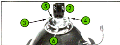
Fig. 7 Projecteurs « CIBIE » 2 - Connecteur 3 - 4 - Ressorts de maintien 5 - Collerette d'ampoule 6 - Ergot de positionnement
