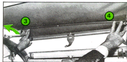
Fig. 32] Ouverture avant de la capote 3 - Cadre 4 - Traverse
