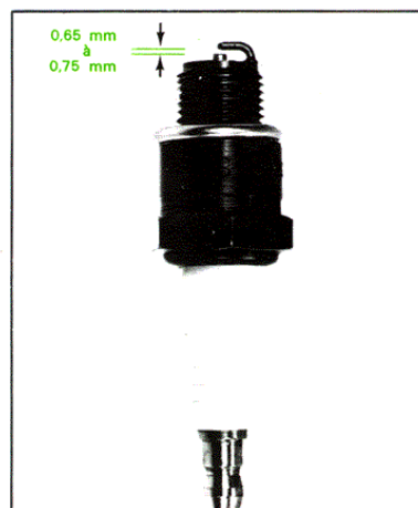
Fig. 12] Bougie : Ecartement des électrodes
