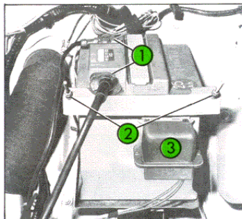
Fig. 11 Batterie 1 - Bornes 2 - Tirants 3 - Régulateur
