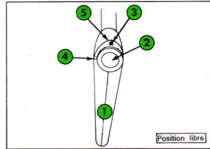
Fig. 20 Frein de secours et d'immobilisation 1 - Poignée de frein 2 - Bouton de sécurité 3 - Taquet de verrouillage 4 - Encoche de blocage du taquet 5 - Encoche de déblocage
